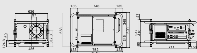
● 外形寸法図
