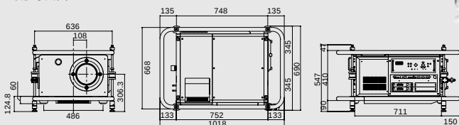
● 外形寸法図
