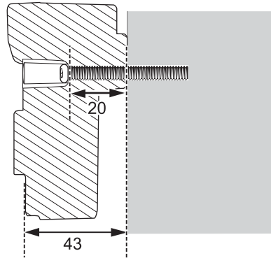
Querschnitt Schraubenloch
